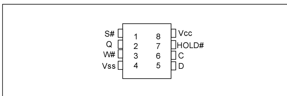
SOP8/TSSOP8/UDFN8
